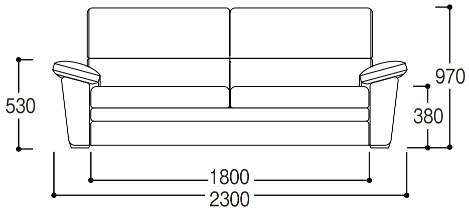
正面図
