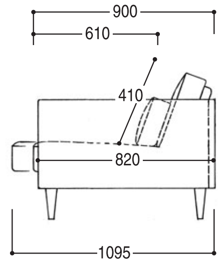
側面図 3.5P
