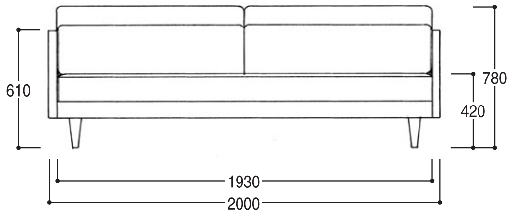
正面図 3.5P
