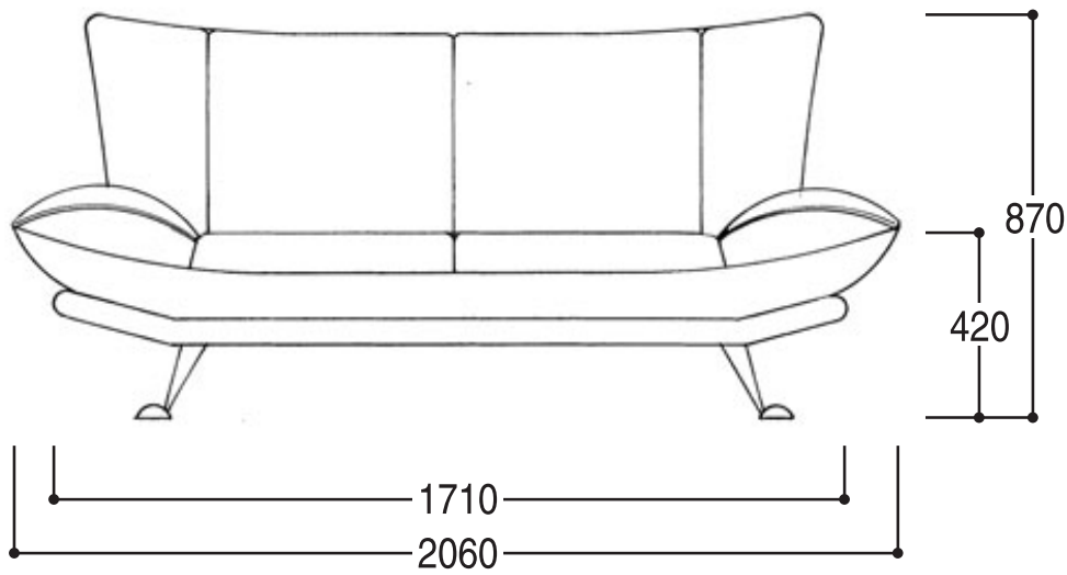
正面図
