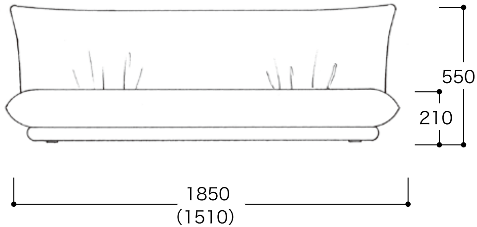
正面図 3P
