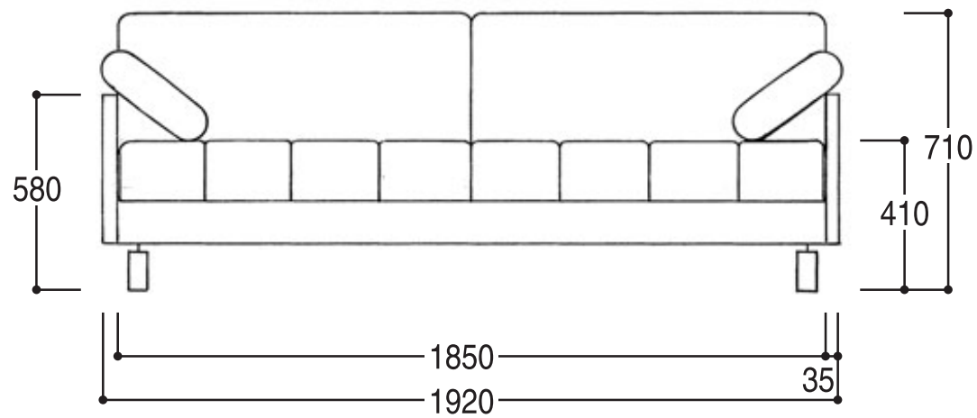
正面图
