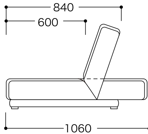
側面図 3P
