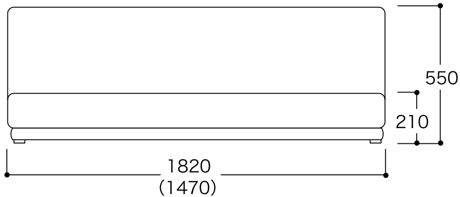
正面図 3P
