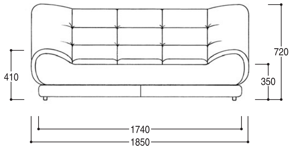
正面図 ケビン(ローバック)
