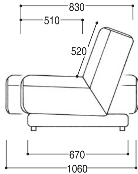
側面図 ケビン(ハイバック)
