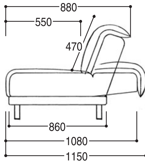
侧面图
