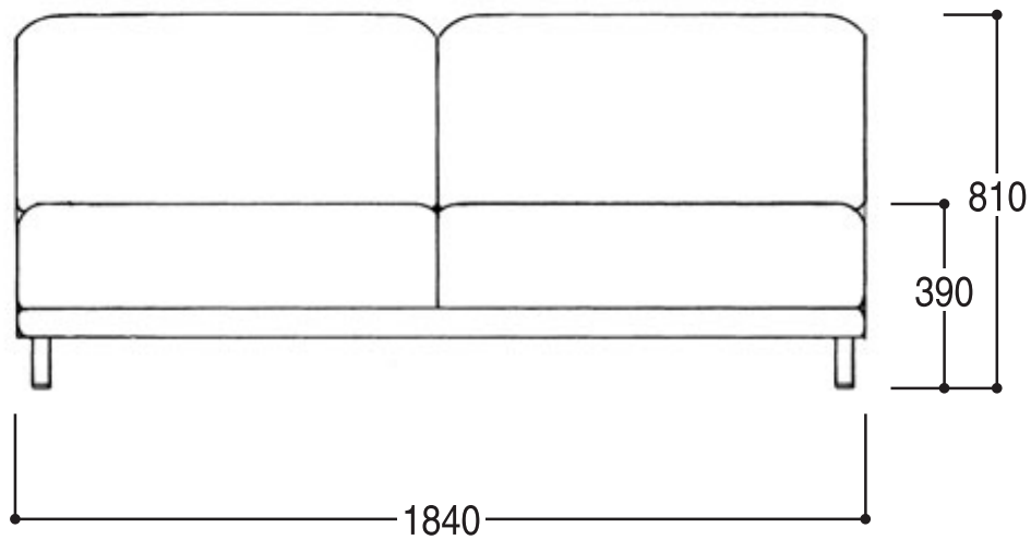
正面图
