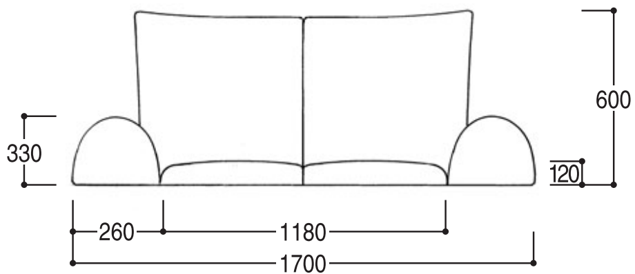
正面図 2P
