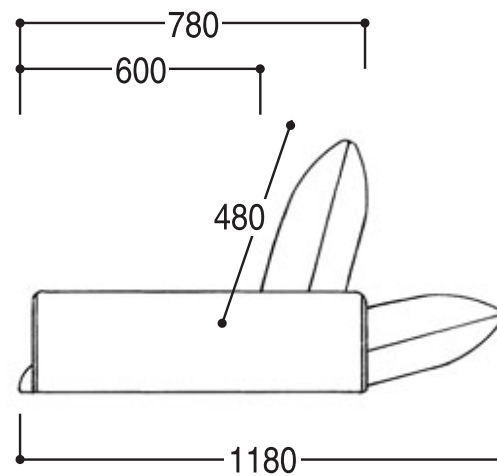
側面図 2P
