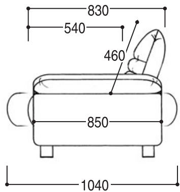
側面図 エブリ
