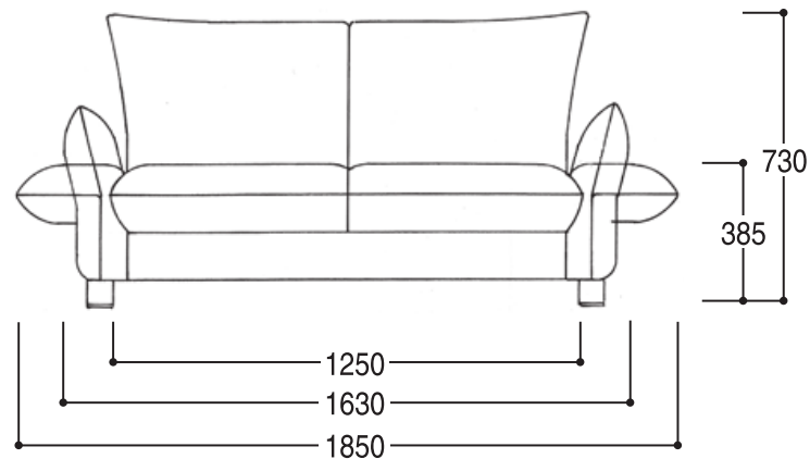
正面図 エブリ 125
