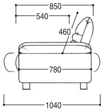
側面図 エバ
