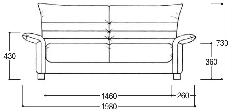
正面図 エバ 145
