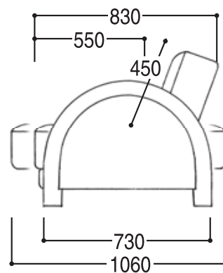
側面図 3.5P 両肘
