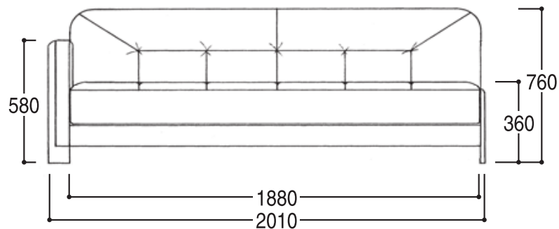
正面図 3.5P 片肘
