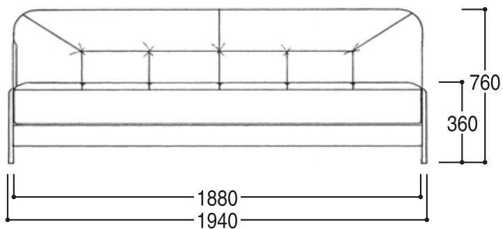
正面図 3.5P 肘無
