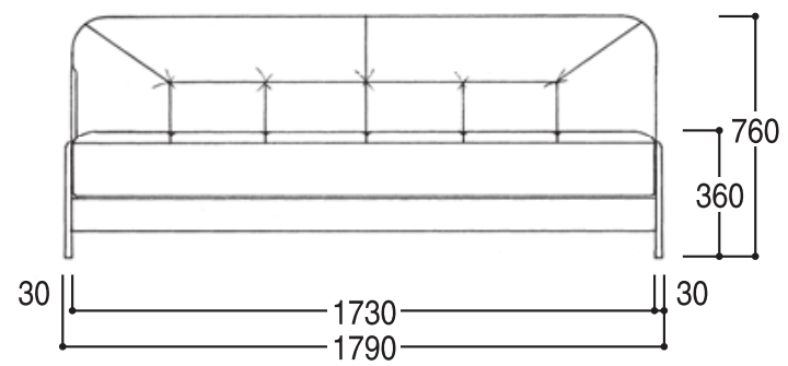
正面図 3P 肘無
