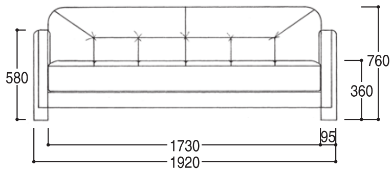
正面図 3P 両肘
