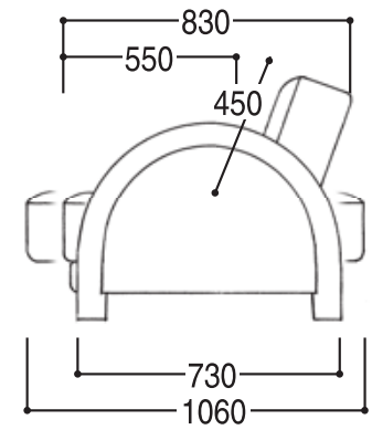
側面図 3P 両肘
