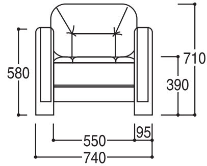
正面图 1P
