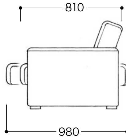
側面図 エポックウッド 1700 / 1900
