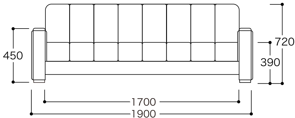
正面図 エポックウッド 1700 / 1900
