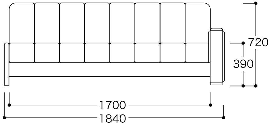
正面図 エポックウッド左肘 1700 / 1840
