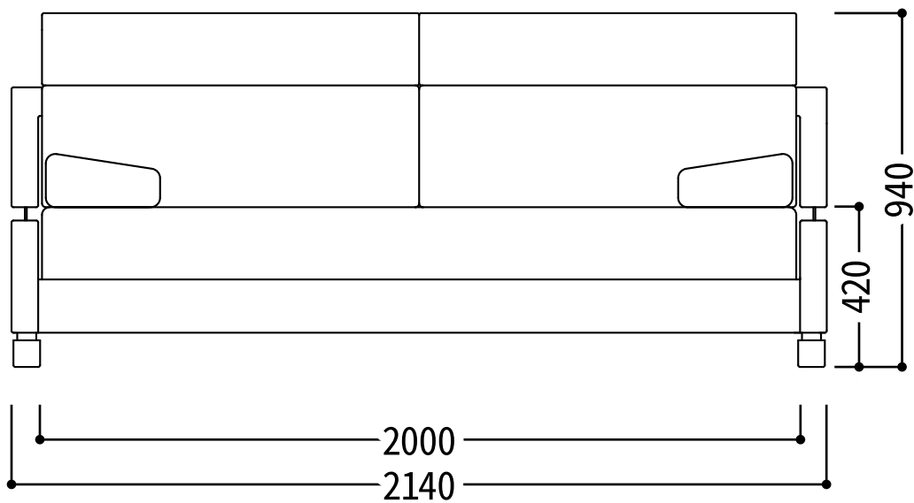
正面图
