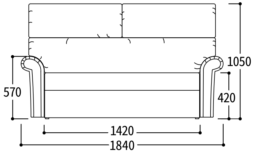
正面図
