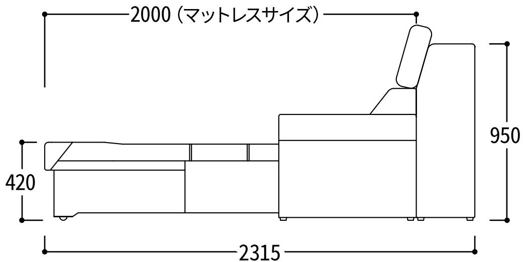
側面図(ベッド)
