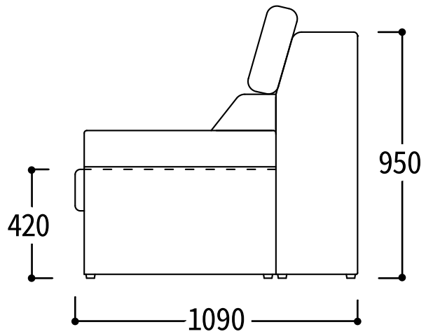
側面図(ソファ)
