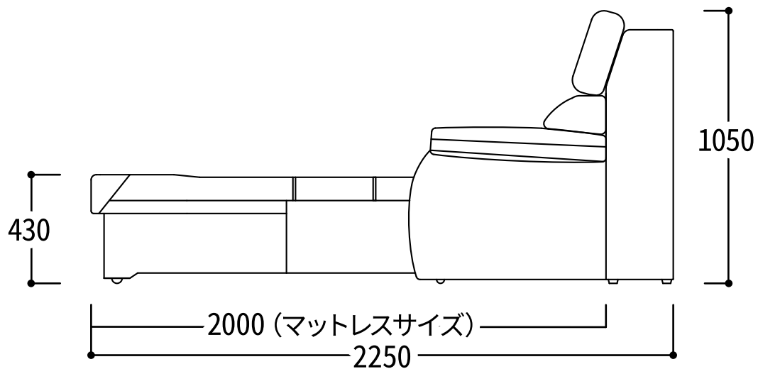
側面図(ベッド)
