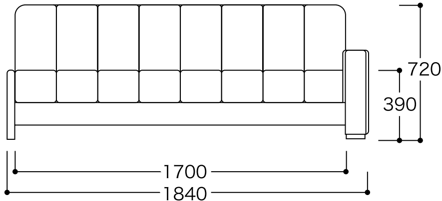
正面図 エポックノン左肘 1700 / 1840
