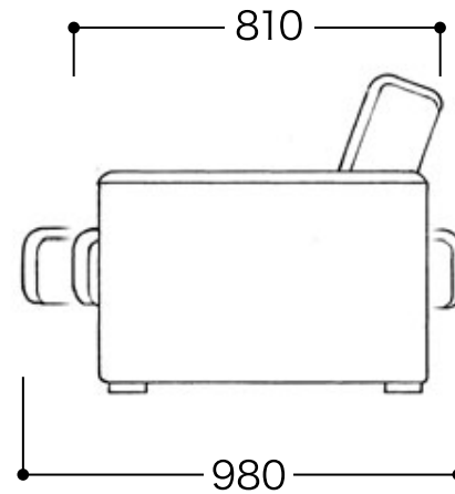
側面図 エポックノン 1700 / 1900
