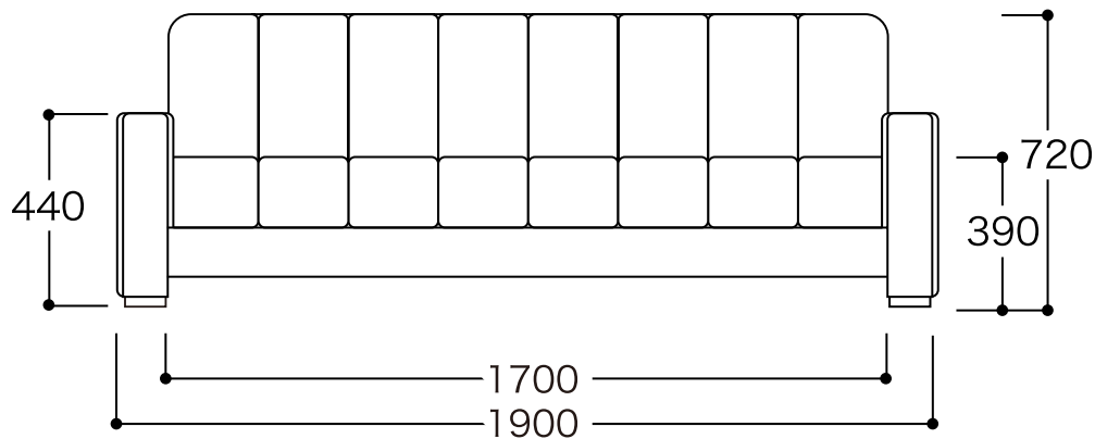
正面図 エポックノン 1700 / 1900
