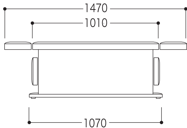
エディ 1000 正面図
