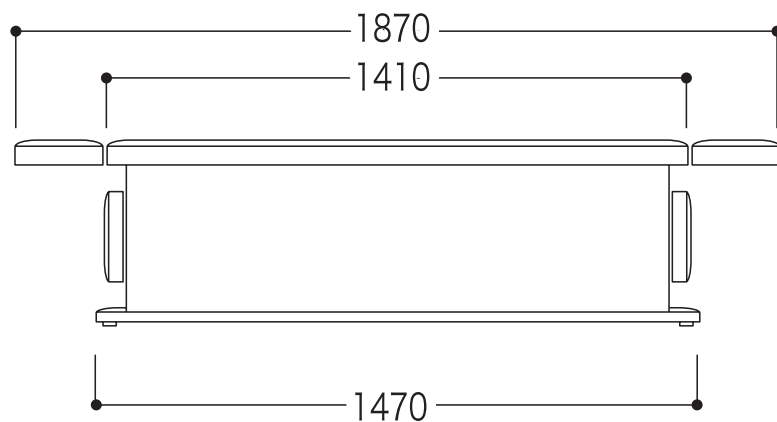
エディ 1400 正面図
