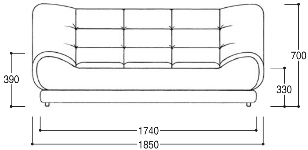
正面図 ドン(ローバック)
