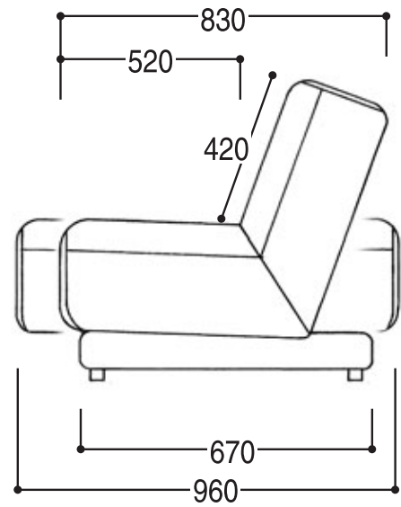
側面図 ドン(ローバック)
