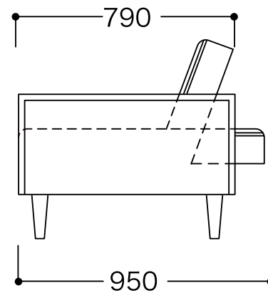
侧面图
