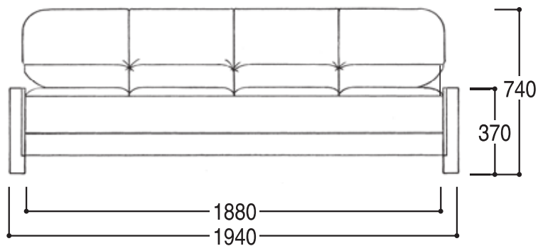
正面図 3.5P 肘無
