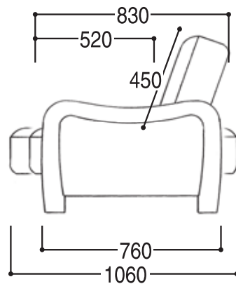
側面図 3.5P 両肘
