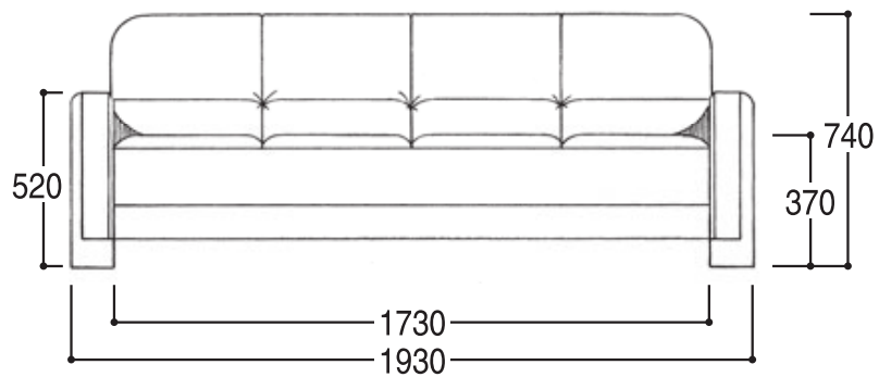
正面図 3P 両肘
