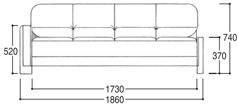
正面図 3P 片肘
