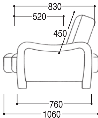
側面図 3P 両肘
