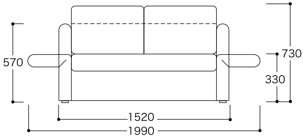
正面图
