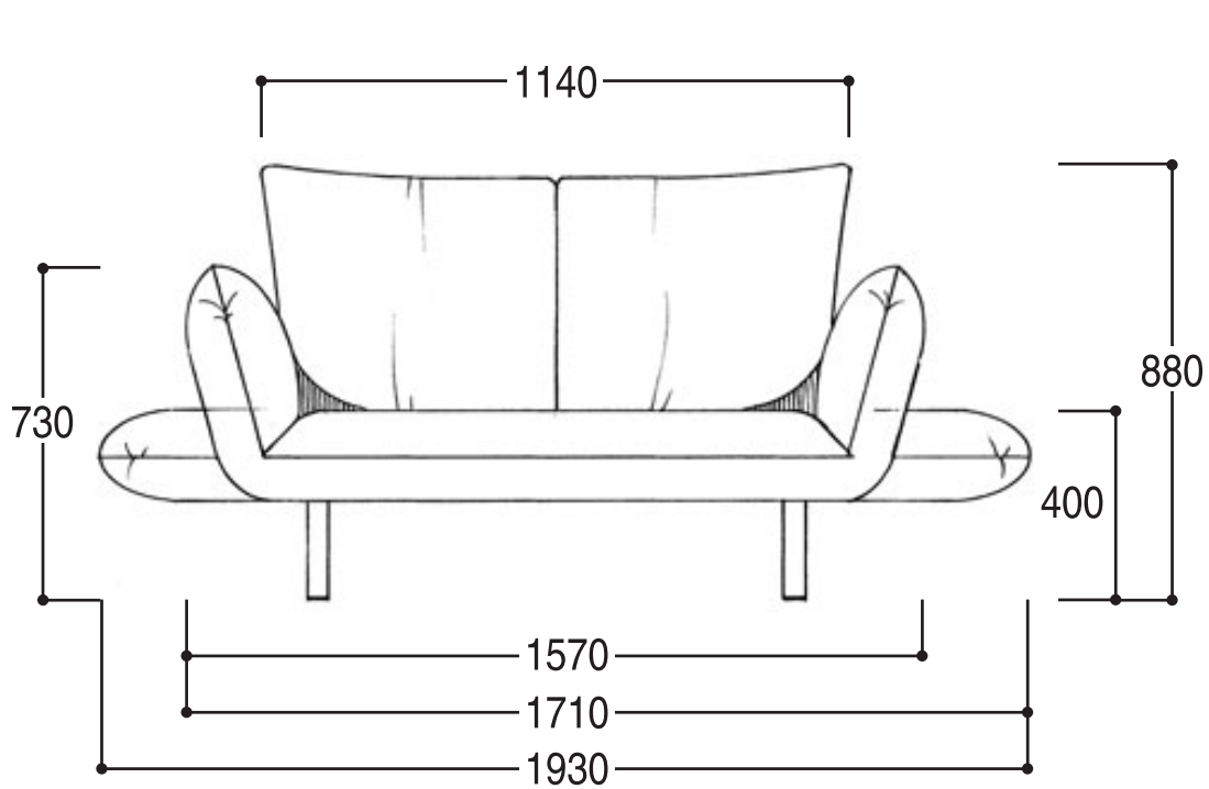
正面图
