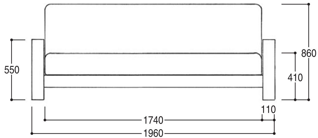
正面図 3P
