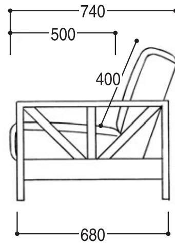
側面図 1P
