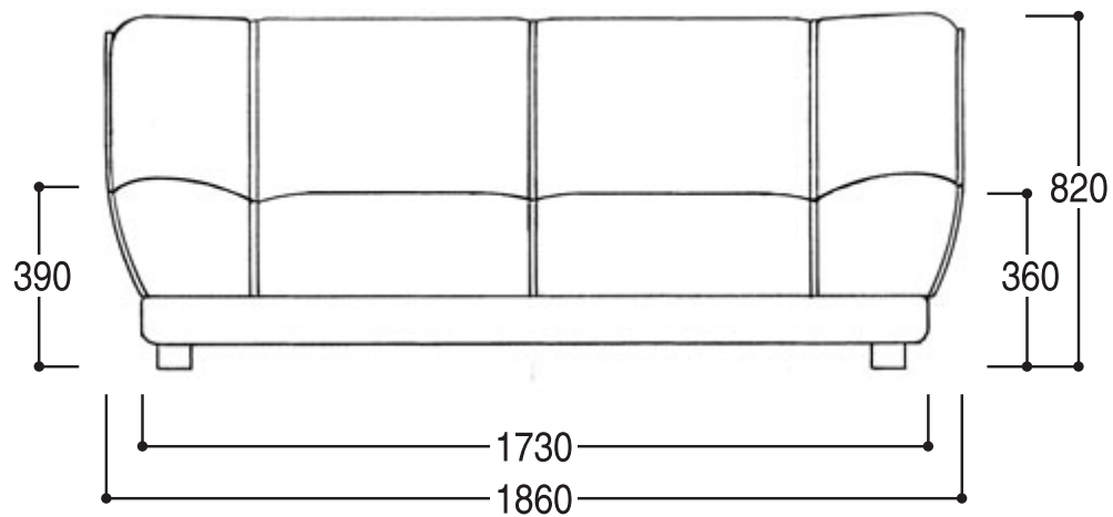
正面图
