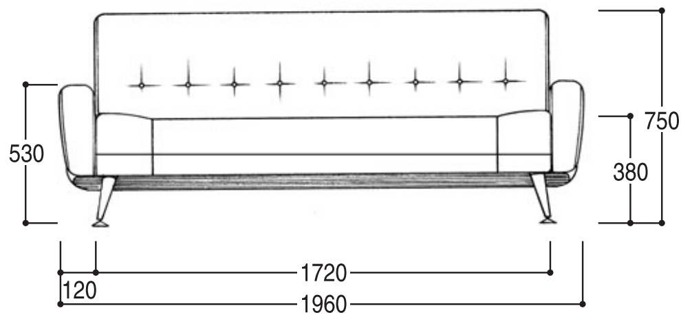
正面图 3P
