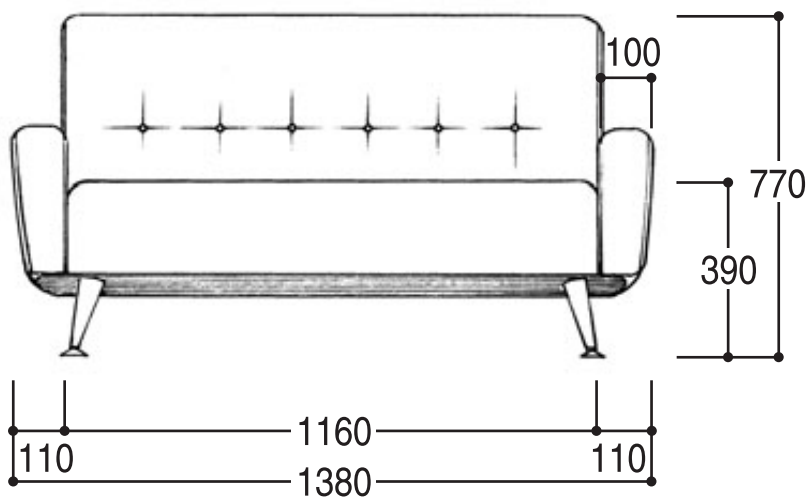
正面図 2P
