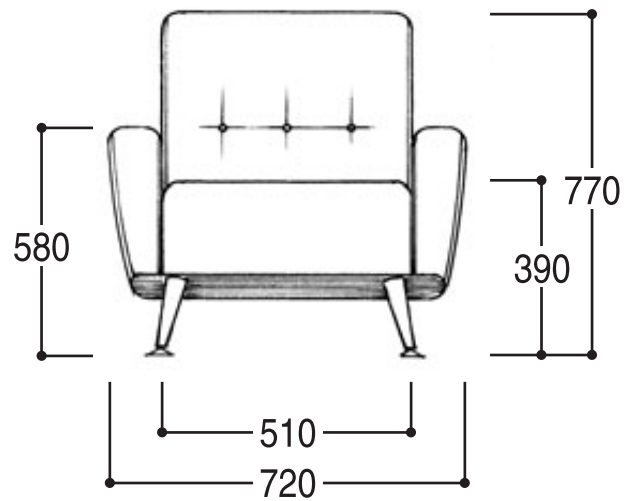
正面图 1P
