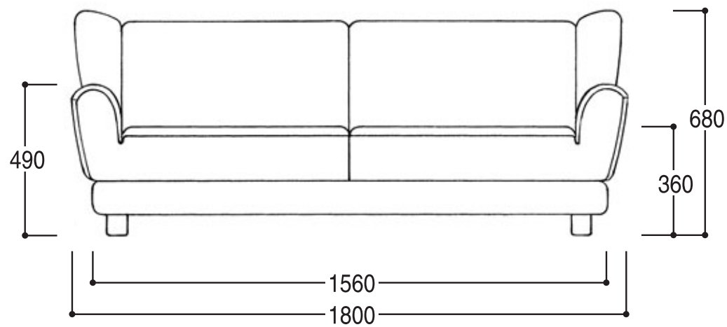
正面图 3P
