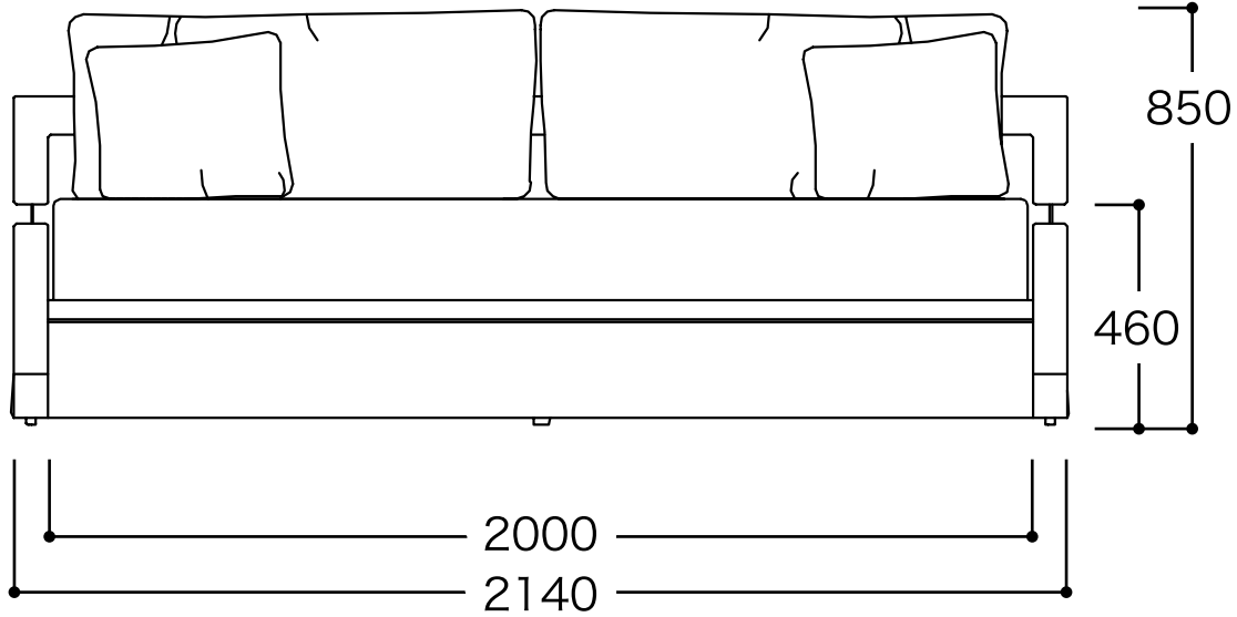
正面图
