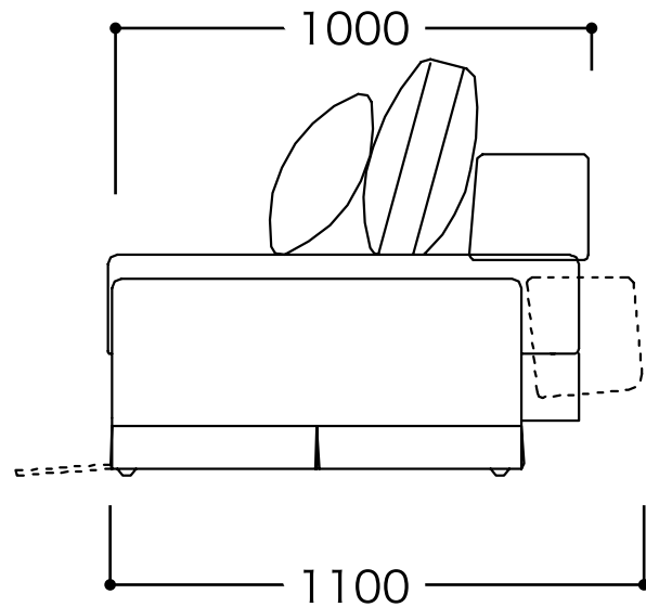
侧面图
