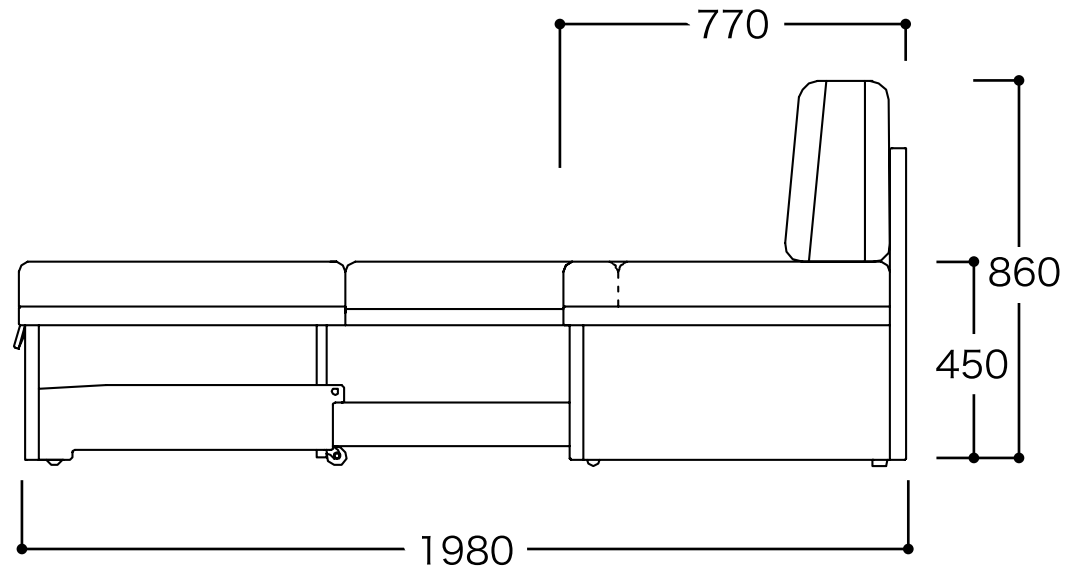
プリア 側面図
