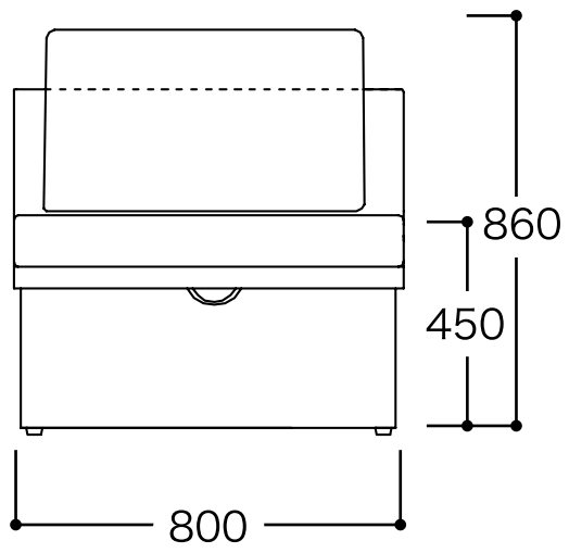
プリア W800正面図
