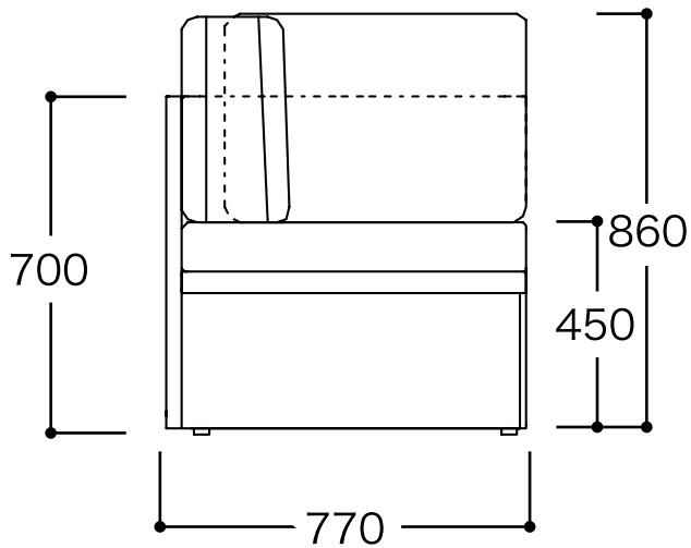
ワニータコーナ 正面図
