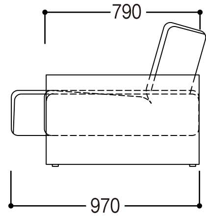
側面図 2040
