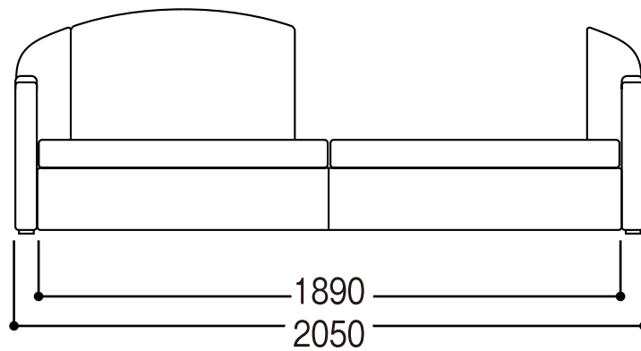
正面図
